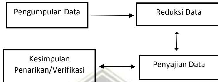
Gambar 3.1 Analisis Data
