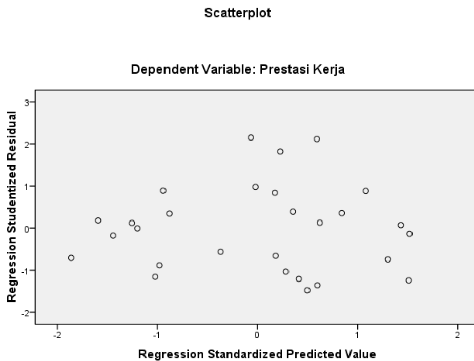
Gambar 4.2 Uji Heterokedastisitas
