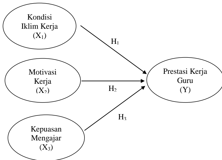
Gambar 2.1 Kerangka Pemikiran
